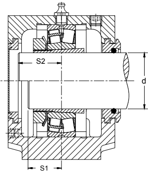
Roulements à alésage conique sur manchon de serrage Disque d'obturation/Joint labyrinthe
