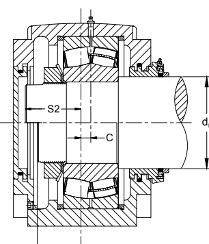
Roulement à alésage cylindrique Disque d'obturation/Joint taconite
